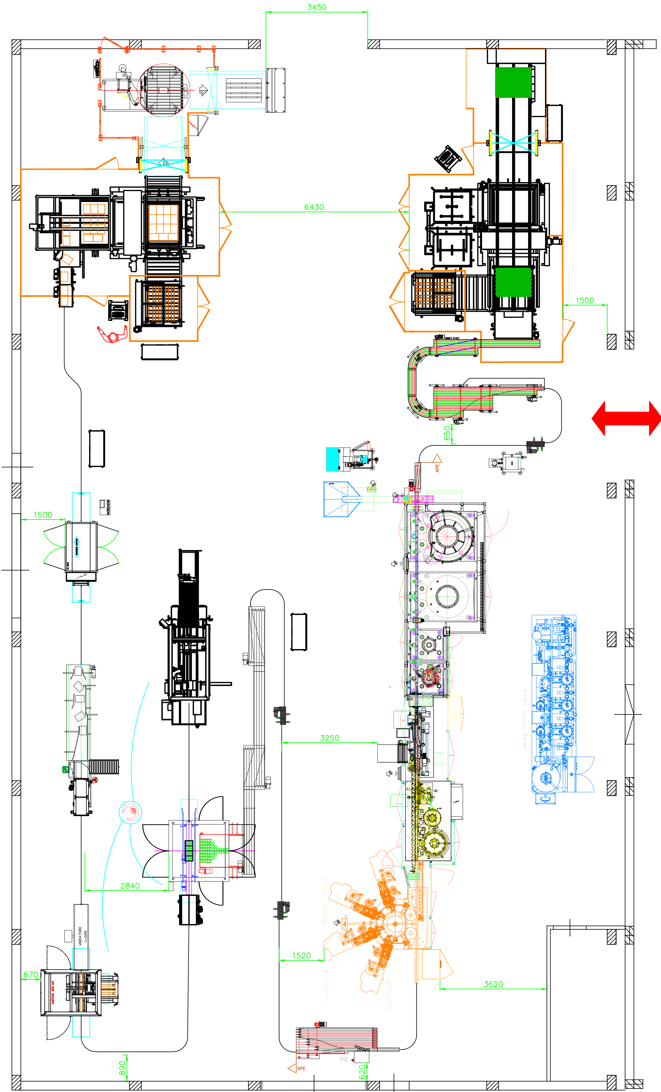
LINEA 10.000 bph
